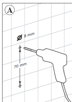
Fissaggio a muro
